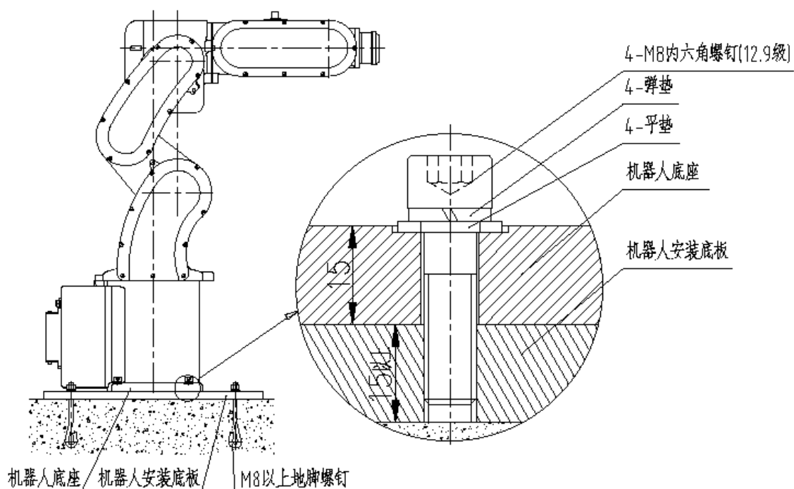
图3 机器人安装举例
