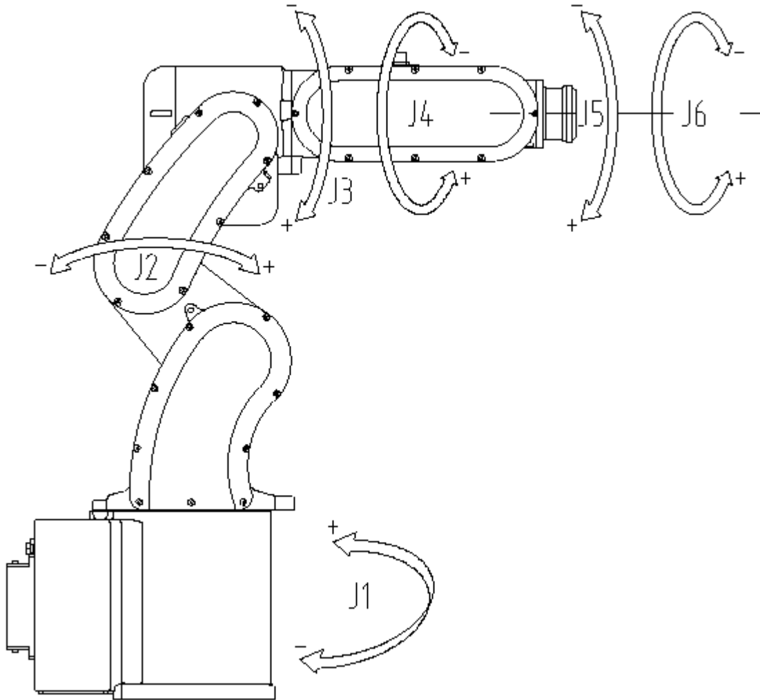
图 6 机器人各轴名称及方向
