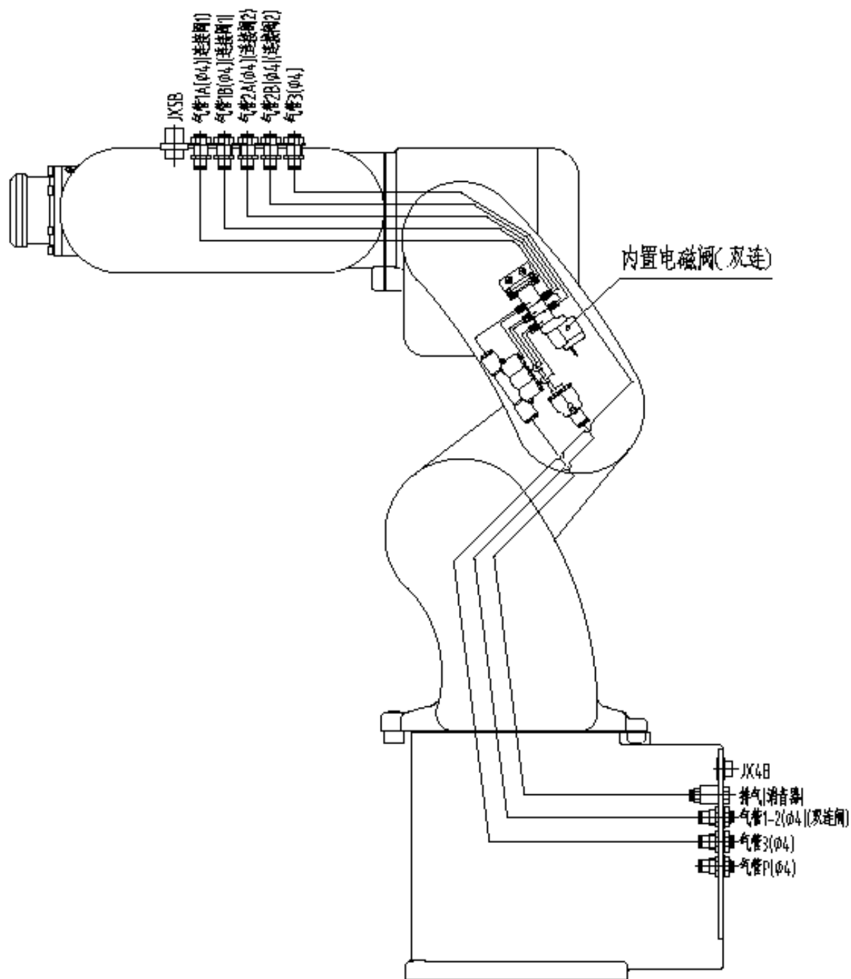
图 11 机器人配管图
