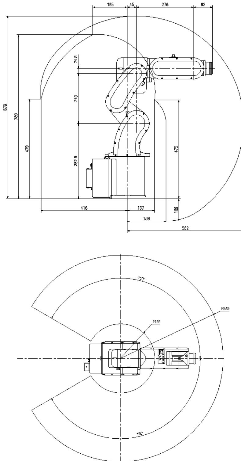
图 10 机器人的最大运动范围
