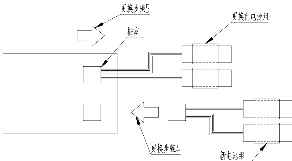
图 13 电池组连接
