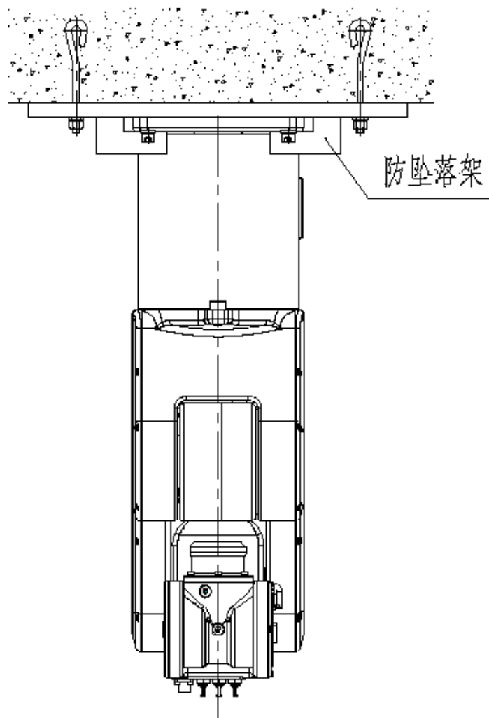
图 5 防坠落方法
