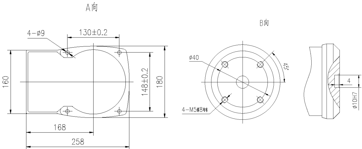
图 7 机器人外形尺寸
